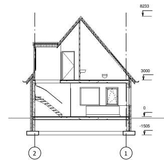
Doorsnede A-A
